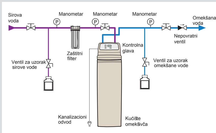
Dijagram - Primer povezivanja Aquaset sistema
